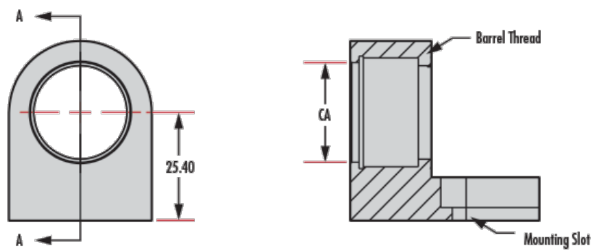
L-Slot Type (#36-410 & #36-416)
