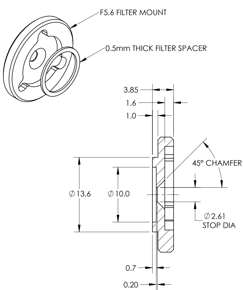
SECTION A-A
