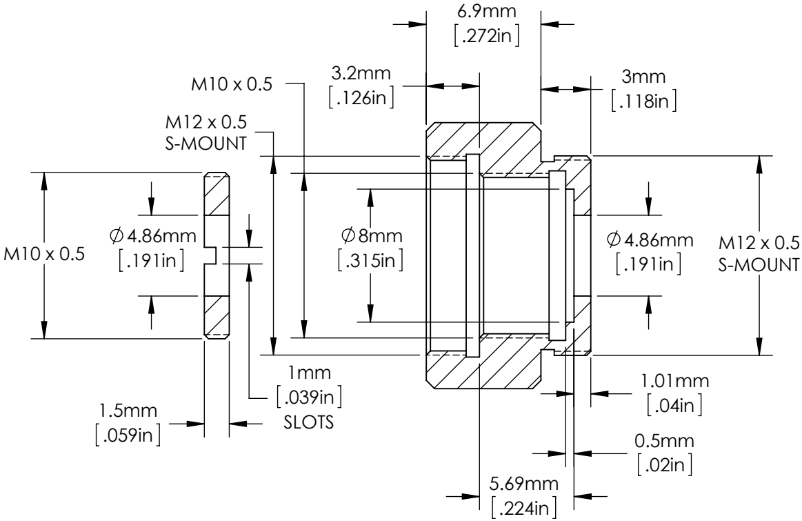
SECTION A-A
