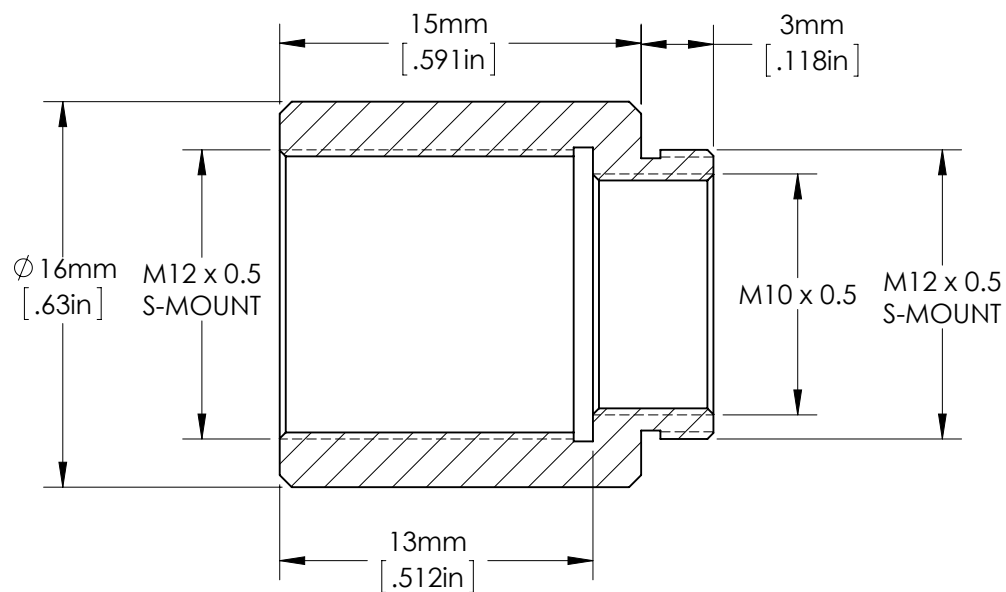
SECTION A-A
